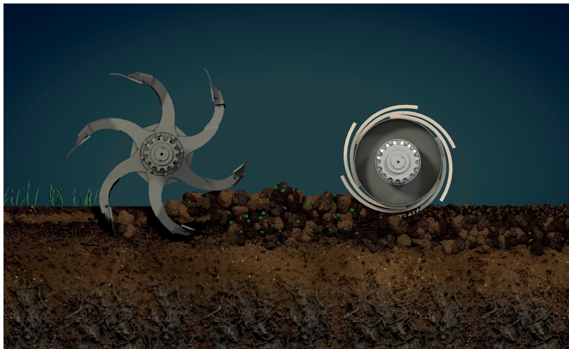
Bewerking van spitas met harkrol
