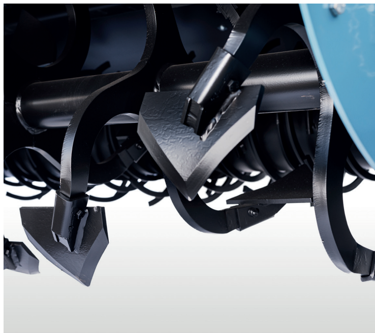
▲ De Eco-Mix spitas
