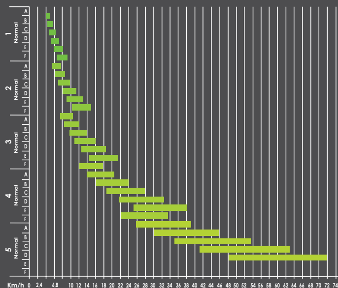
Nieuwe RCShift-transmissie, volledig gerobotiseerd en elektronisch afgesteld op 50 km/u, waar wettelijk toegestaan.
